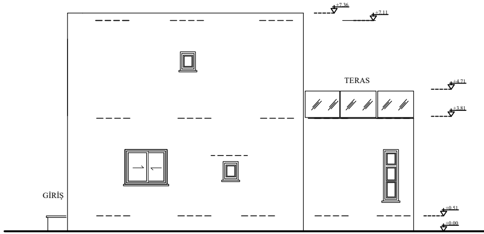
GÜNEY CEPHESİ ÖL:1/100
