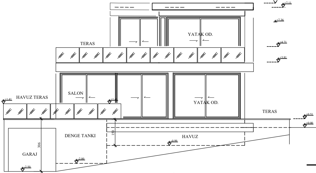
KUZEY CEPHESİ ÖL:1/100
